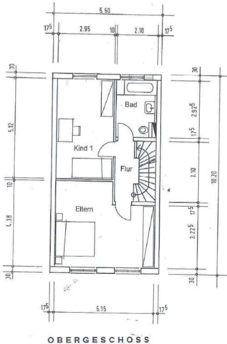
Grundskizze OG
