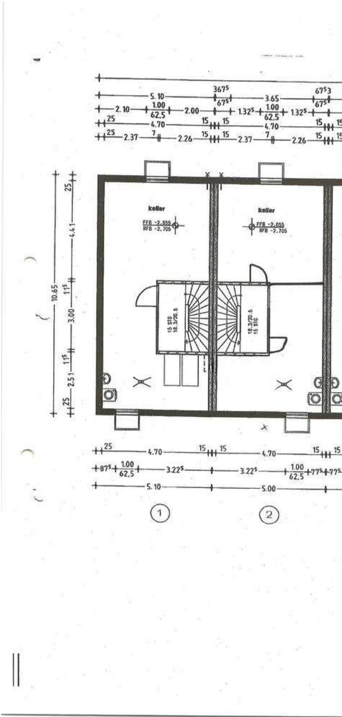
Kellergeschoss
